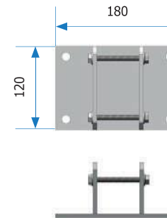
Fijación a suelo alornillado 180x120mm
