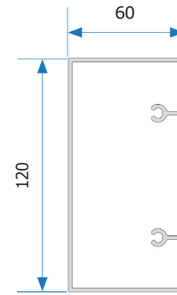
Pgrfil viga 120x60mm
