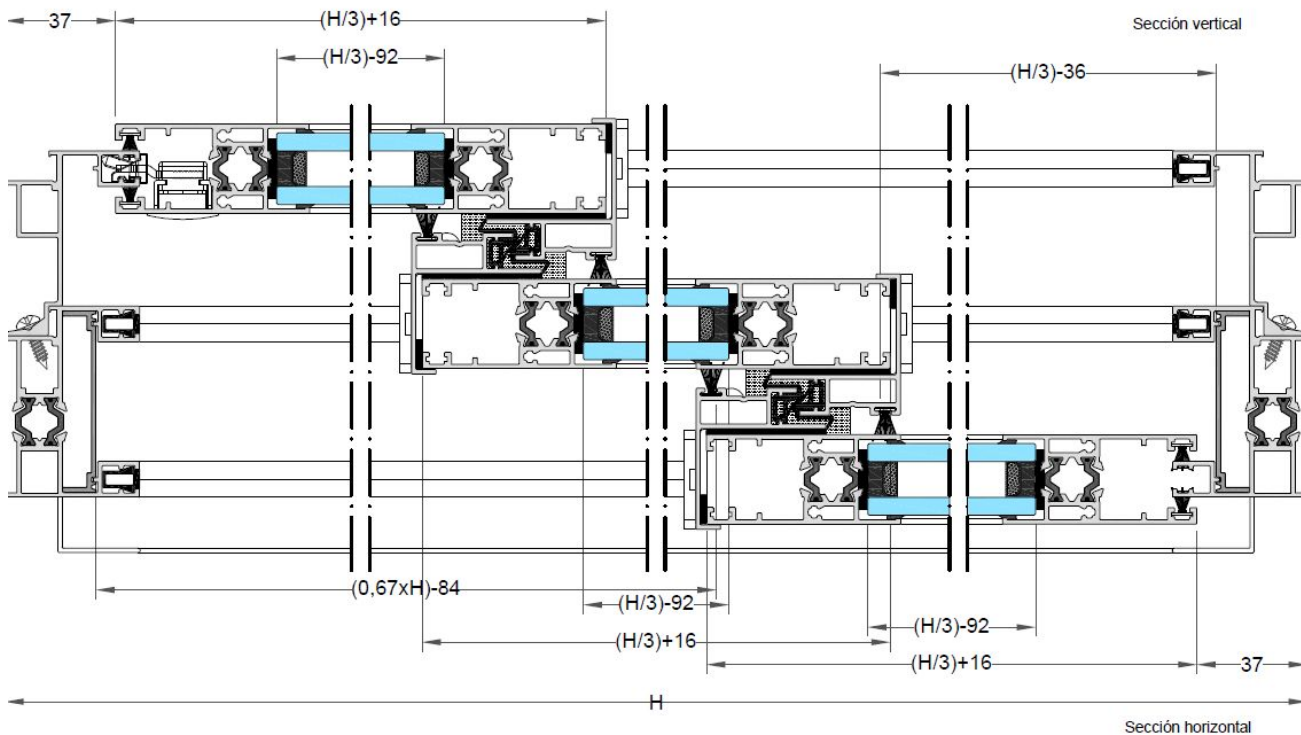
Sección horizontal
