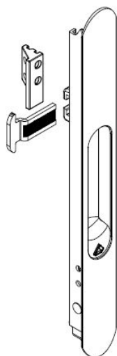
Cierre embutido Ref.: H09031
