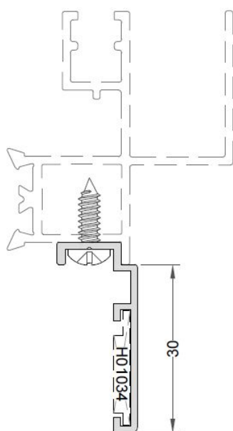
Solape resalte 30 Ref.: 9430
