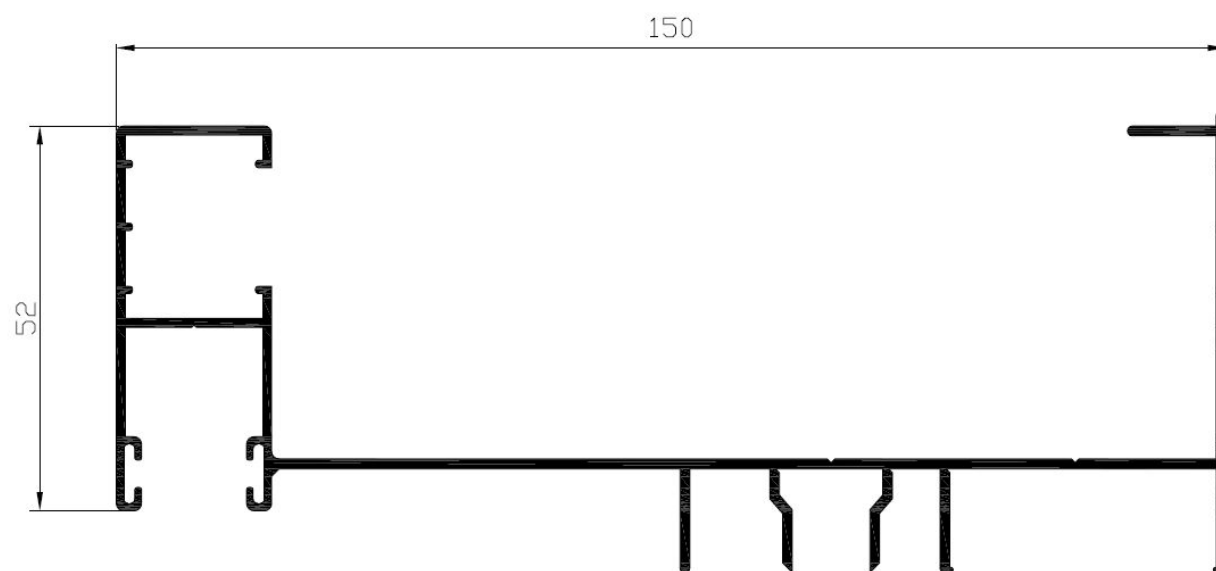
Marco lateral izquierdo con guía Ref: 7054 (INTEGRAL)
