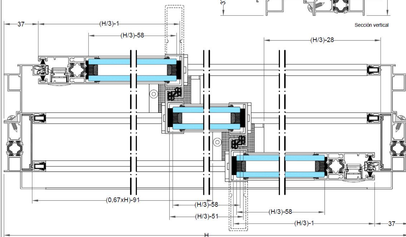
Sección horizontal
