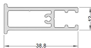
Unión 4 hojas Ref.: 8410
