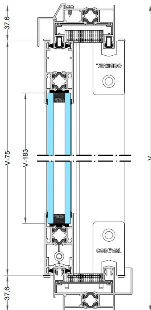
Sección vertical
