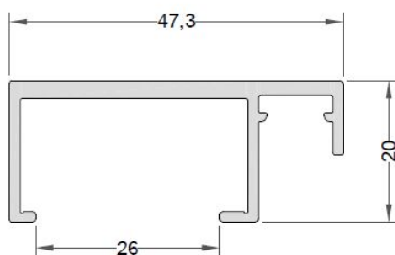
Perfil cruce Ref.: 8415
