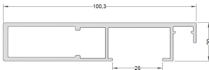
Perfil tirador cruce Ref.: 8405
