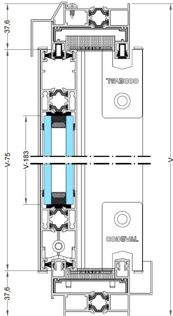
Sección vertical
