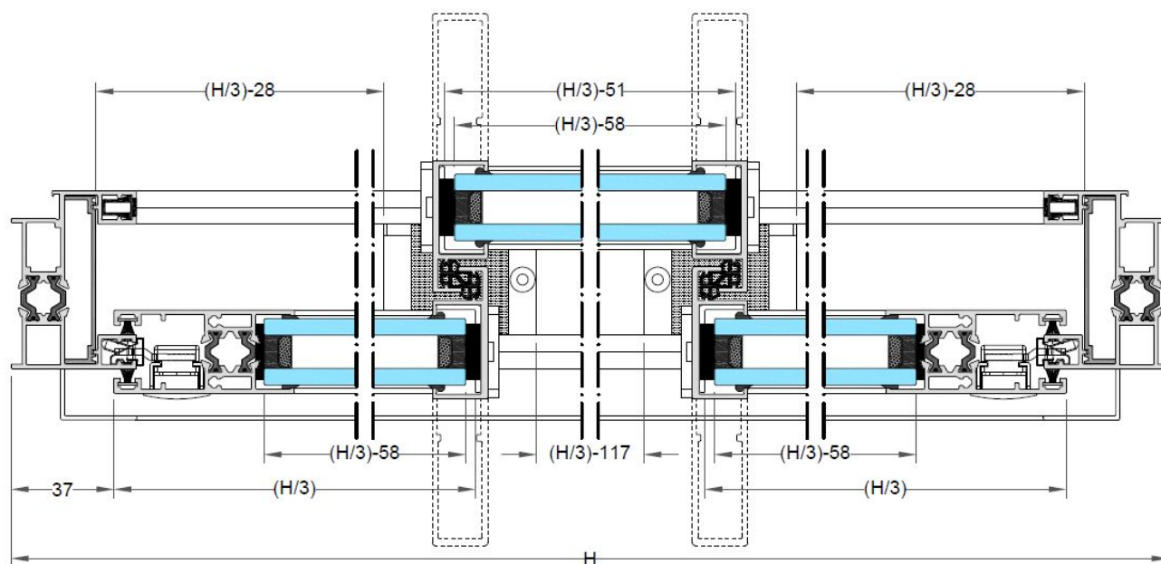
Sección horizontal
