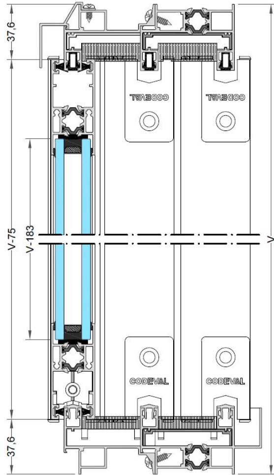
Sección vertical
