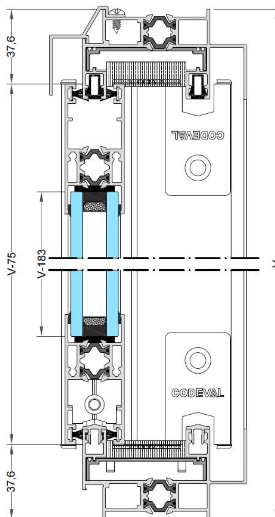
Sección vertical
