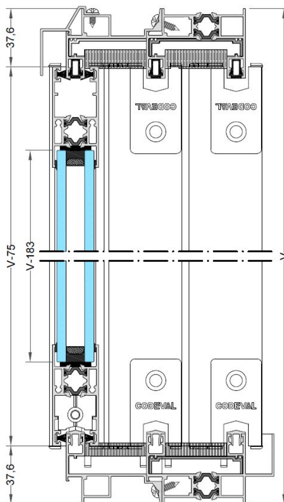
Sección vertical
