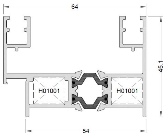
Marco liso Ref.: 8401
