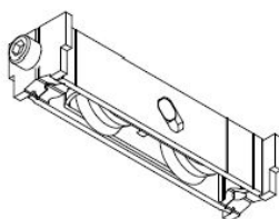
Rodamiento TANDEM regulable (160 Kg/hoja) Ref.: H32034
