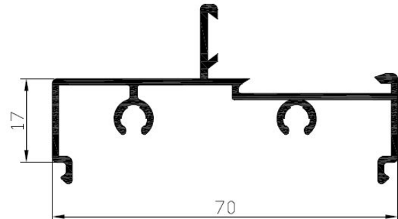
Marco fijo c.clip Ref: 7011
