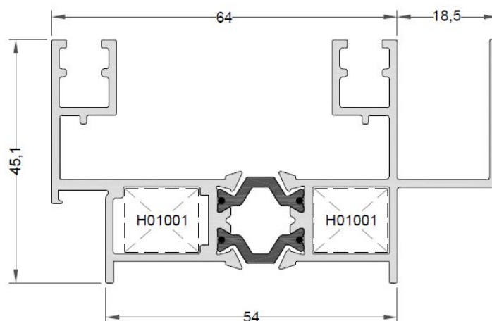
Marco con vierteaguas Ref.: 8402
