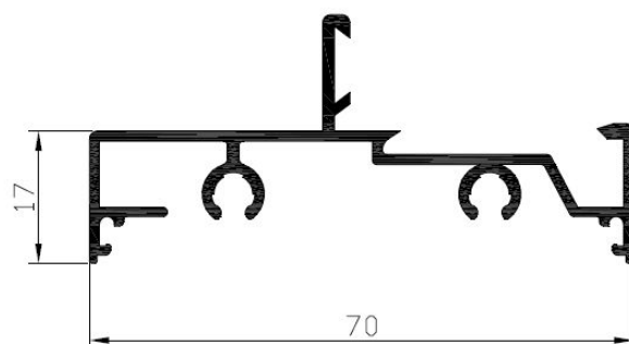
Marco fijo s.clip Ref: 7012
