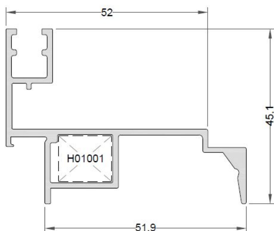
Marco tercer carril Ref.: 8403
