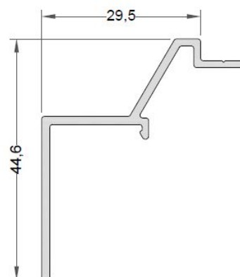
Vierteaguas exterior Ref.: 8419
