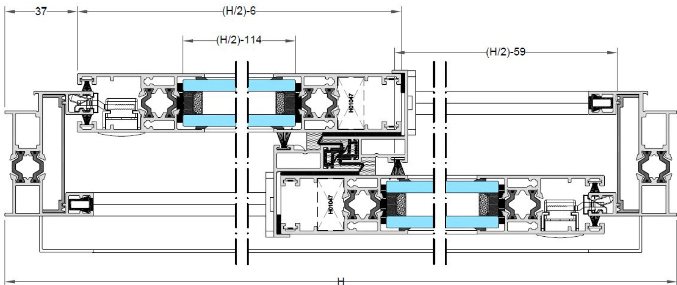
Sección horizontal
