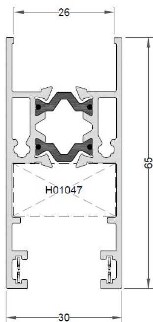
Hoja hueco 26 Ref.: 8414
