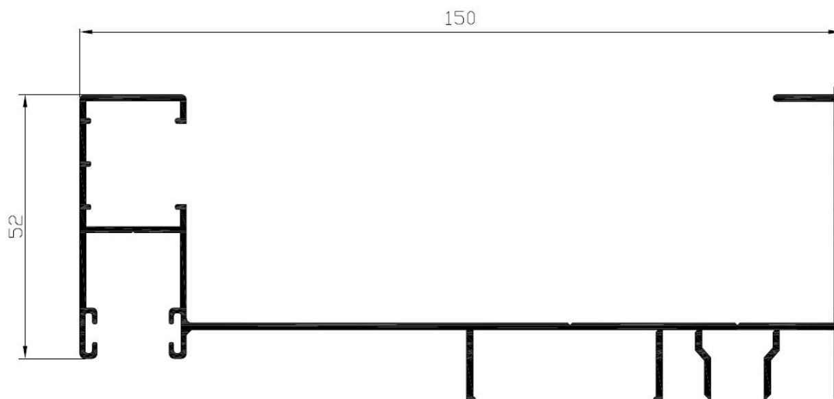
Marco lateral derecho con guía Ref: 7044 (INTEGRAL)
