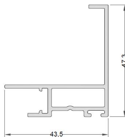
Clip hoja central perimetral Ref.: 8425
